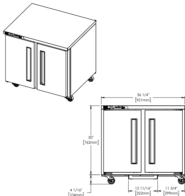
ELEVATION
