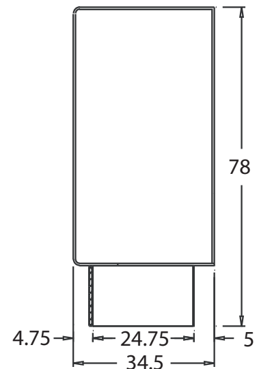
OD35E SOLID SIDE STANDARD
