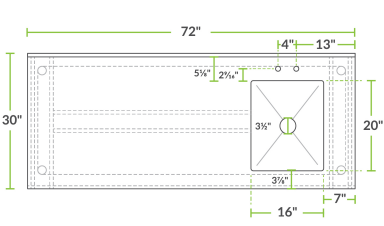
TOP
