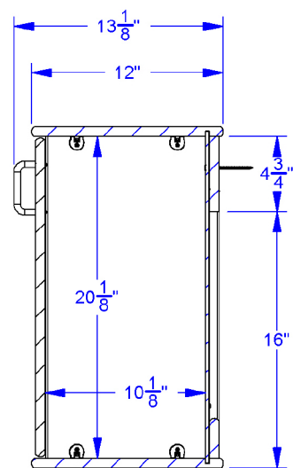
SECTION A-A
