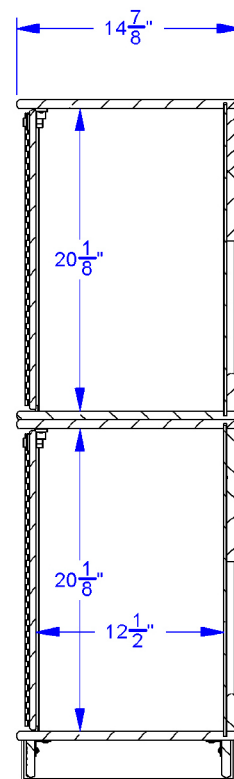
SECTION A-A
