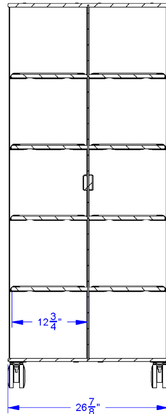
SECTION A-A
