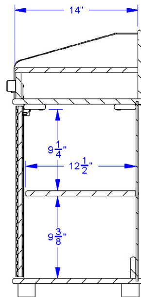
SECTION A-A
