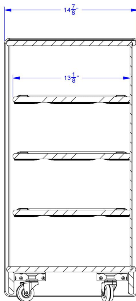
SECTION A-A
