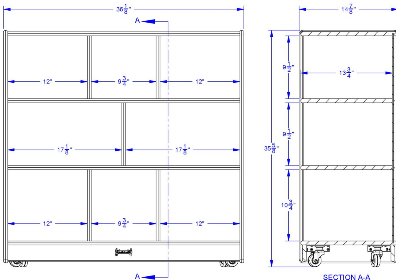
SECTION A-A
