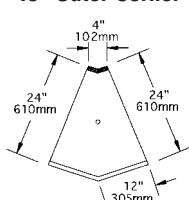
model #WBOC45-24
