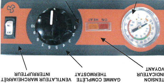
(Fig. 6) THERMOMÈTRE VOYANT INDICATEUR DE CHALEUR
