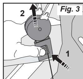
Languette de la plaque de maintien
