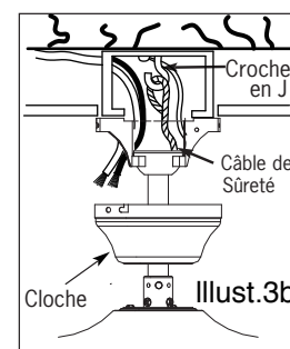
Vis de la boîte électrique (en sus)
