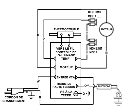
DIAGRAMME DE CONNEXION
