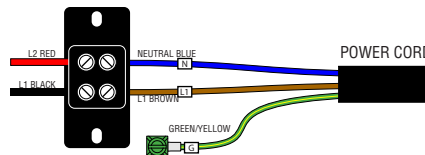
230 volt ac models
