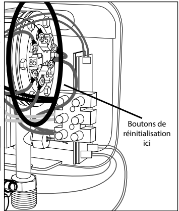
Figure 26 - Emplacement des boutons de réinitialisation
