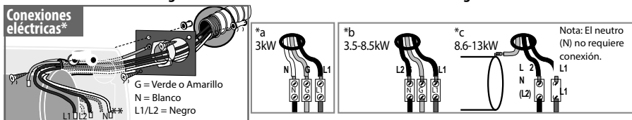
Figure 39 - Detalle de las conexiones eléctricas del calentador de agua
