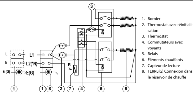
Figure 24 - Câblage du chauffe-eau
