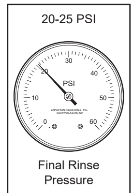
Fig. 19 - Gauge Face
