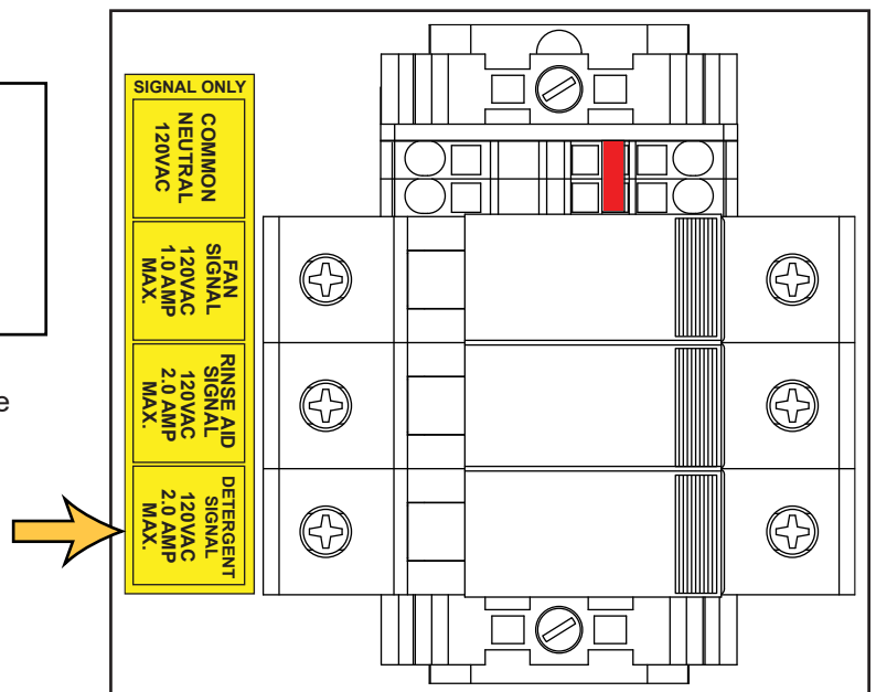
Fig. 27 - Vent fan signal connection
