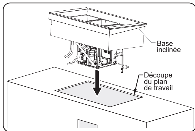
Installation d'une base inclinée
