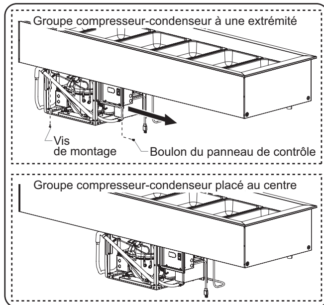
Déplacement d'un groupe compresseur-condenseur
