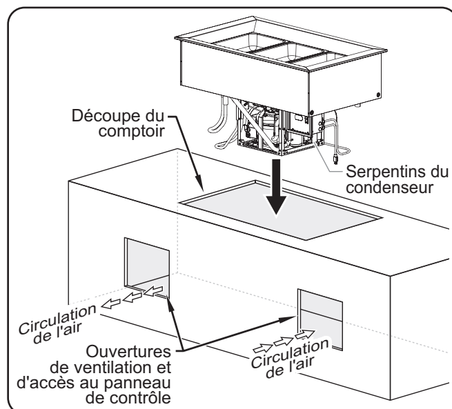
Installation d'un modèle CWB-3
