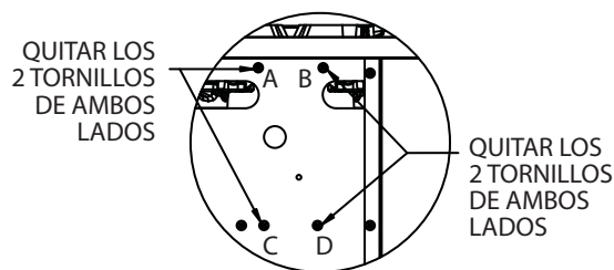
DETALLE II PARA COCINAS DE 60" CON HORNO CONVENCIONAL
